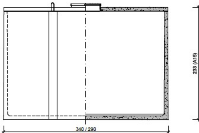
VOORAANZICHT / DOORSNEDE VUE FRONTALE / COUPE
